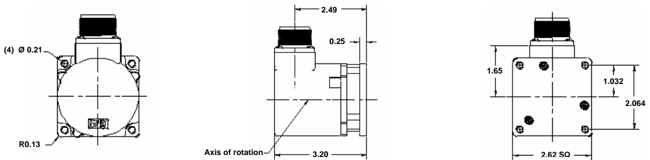
ES25 Dimensions
